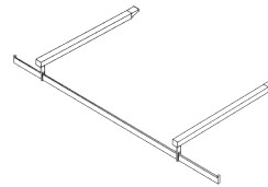
7BAP Barra appenderia con tubo appenderia sotto al ripiano completo di reggi mensola in metallo finitura cromo lucido. Vetro escluso. Crossbar complete with brackets for shelf. In metal in chrome finishing. Glass not included L.115xP.31cm
